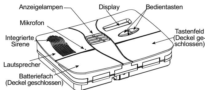
Abb. 1. Funkalarmzentrale mit geschlossenem Deckel
