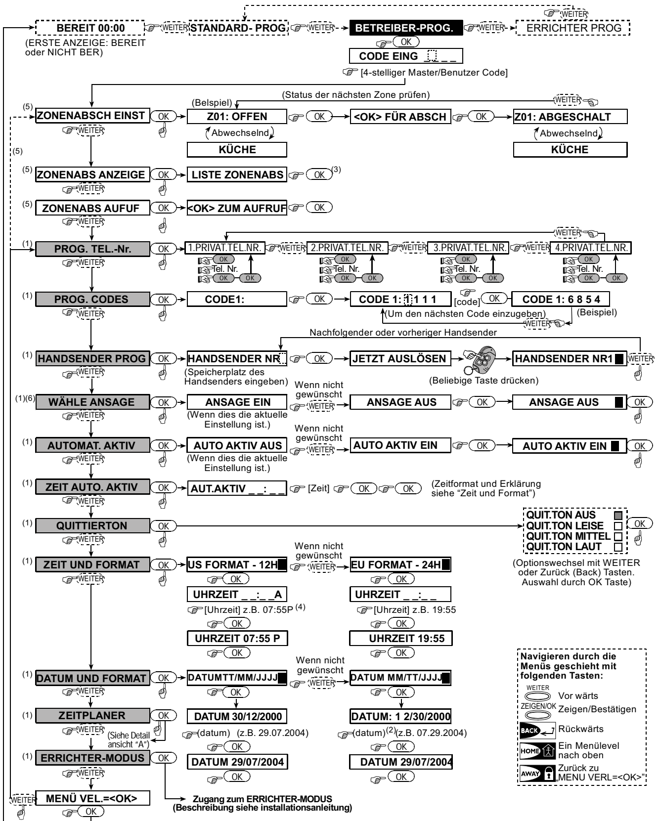
Abb. 8. Ablaufdiagramm „Benutzereinstellungen“
