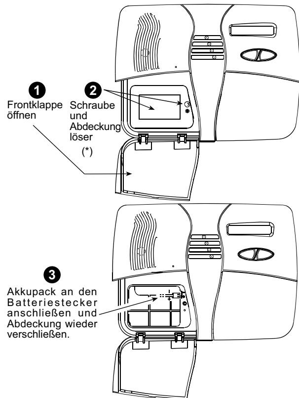
Abb. 10. Batterieerweiterung
