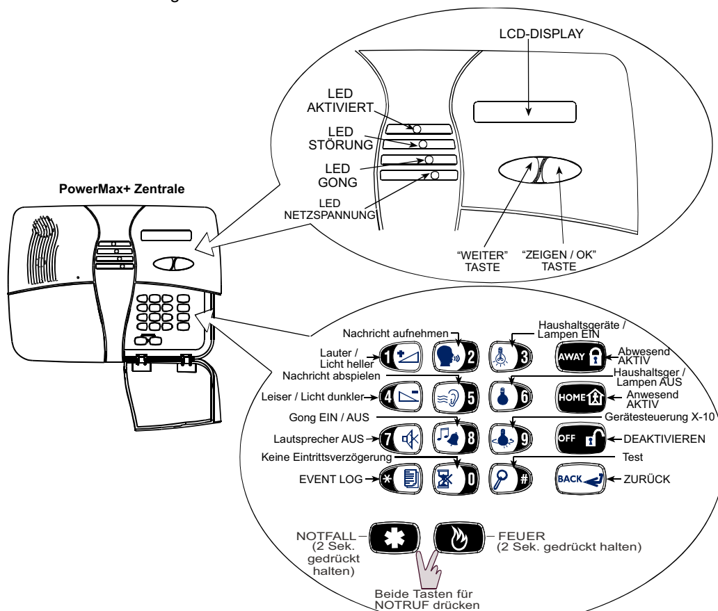
Abb. 4. Bedien- und Anzeigeelemente
