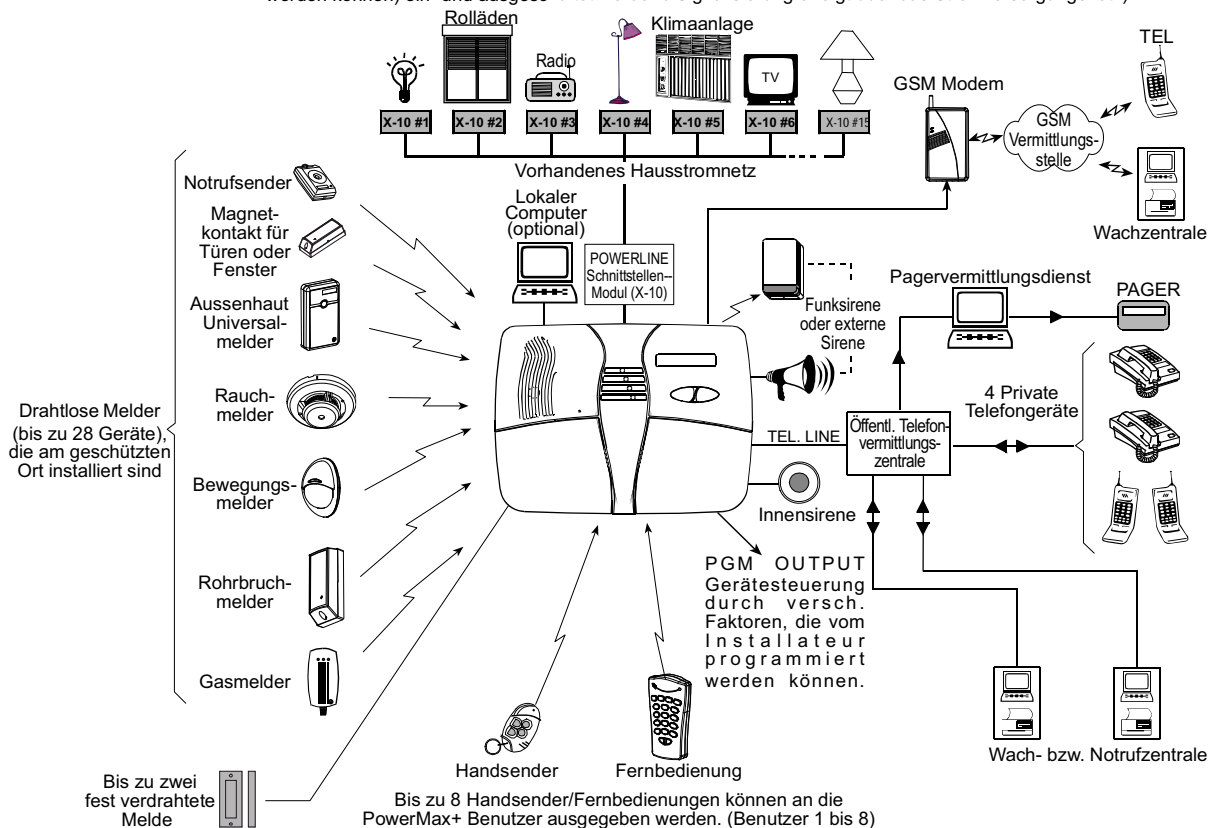
Abb. 2. Typische Systemkonfiguration
